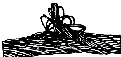
Рис. 10. Выдавливание сердечника
